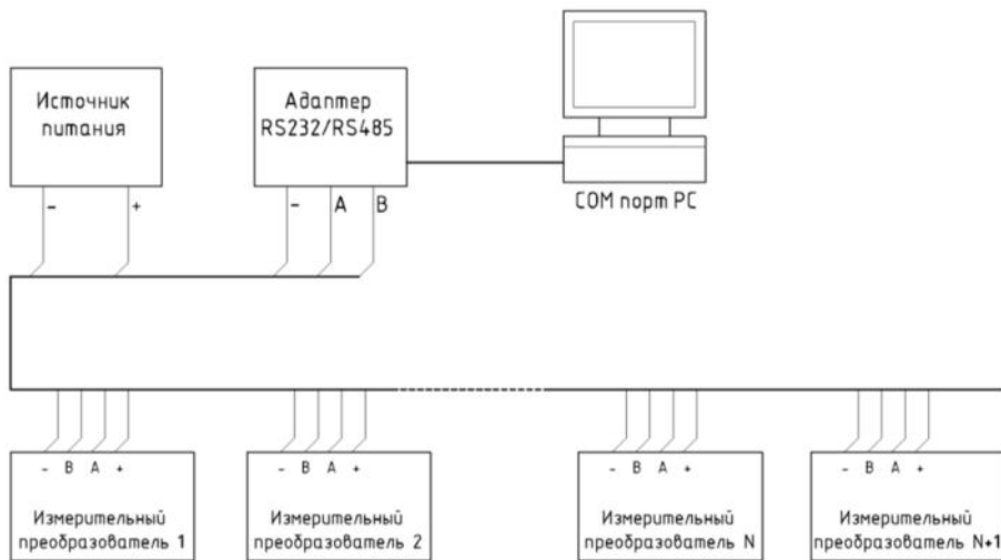
Рис.7. Схема подключения измерительных преобразователей.
