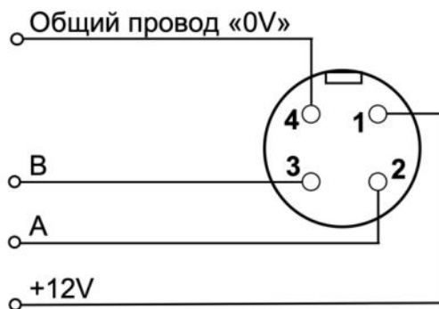
Рис.4. Схема «распайки» кабеля (вид со стороны «распайки» розетки) для подключения ДВ2ТС-5Т-5П-АК исполнение 2.
