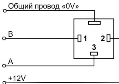
Рис.5. Схема «распайки» кабеля (вид со стороны «распайки» розетки) для подключения ДВ2ТС-5Т-5П-АК исполнение 3.
